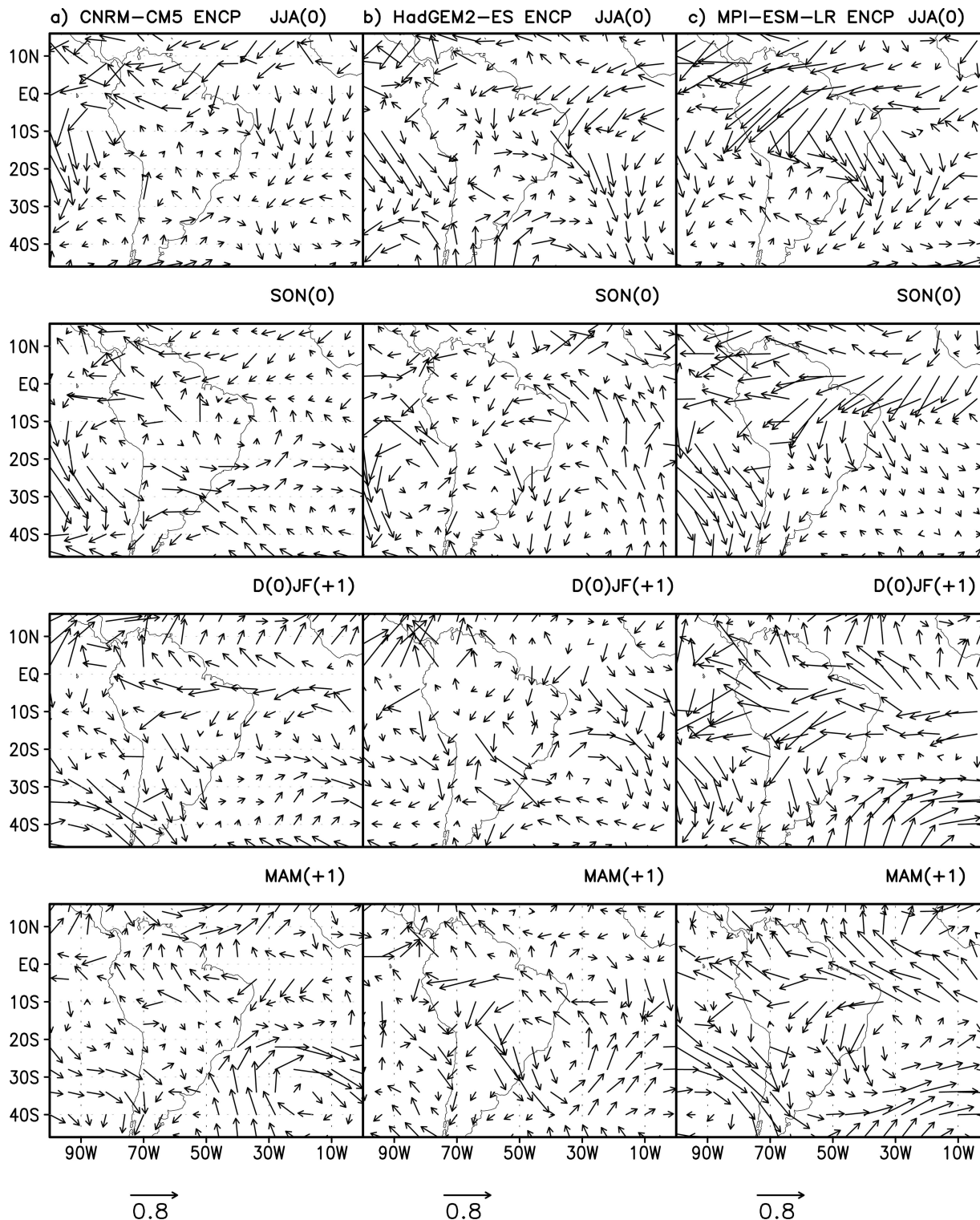
Figura 10 - Composições sazonais de anomalias do vento em 850 hPa de JJA (0) a MAM (+1) para os eventos de EN CP: a) modelo CNRM-CM5; b) modelo HadGEM2-ES; c) modelo MPI-ESM-LR.
