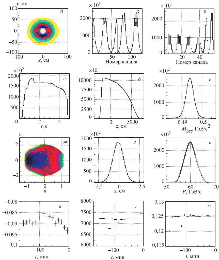
Рис. 2. Примеры гистограмм, формируемых системой мониторинга: а) загрузка одной из дрейфовых камер; б) счетчик срабатываний каналов годоскопа; в) счетчик срабатываний каналов мюонного детектора; г) распределение записанных событий по времени внутри сброса; д) распределение z -координат реконструированных вершин; е) восстановленная масса заряженного каона; ж) распределение событий K_{3\pi}^{\pm} по кинематическим переменным; з) профиль пучка в x -плоскости; и) импульсный спектр пучка; к) временная зависимость x -положения пучка; л) временная зависимость выхода событий K_{3\pi} за сброс; м) временная зависимость доли реконструированных K_{3\pi} среди записанных событий
