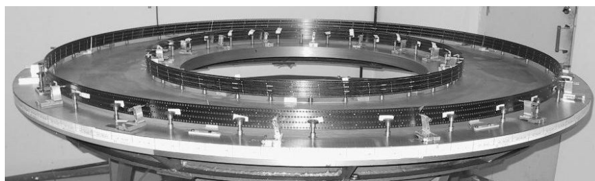
Рис. 4. Кольца внутреннее (В1) и внешнее (В2), подготовленные к установке в них строу
