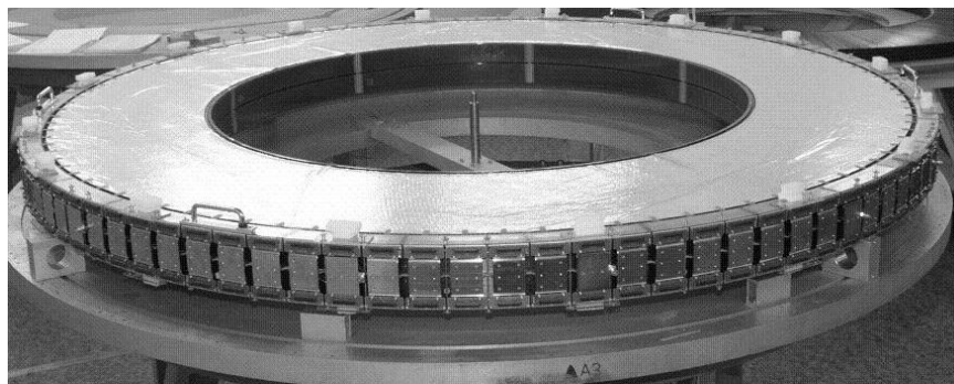
Рис. 1. Внешний вид восьмислойного модуля
