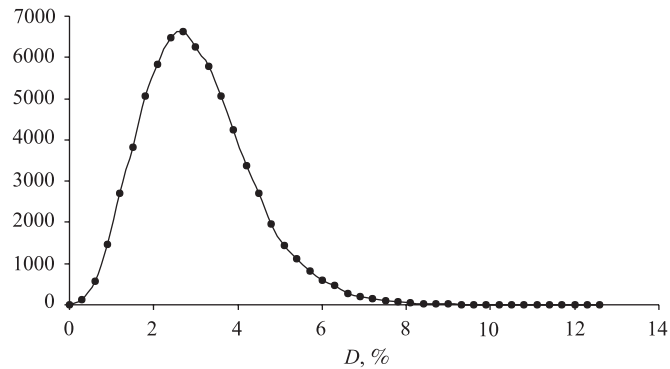
Рис. 7. Распределение величины D , характеризующей однородность газового усиления в строу
