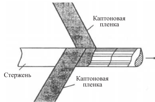
Рис. 2. Схематическое изображение процесса намотки строу
