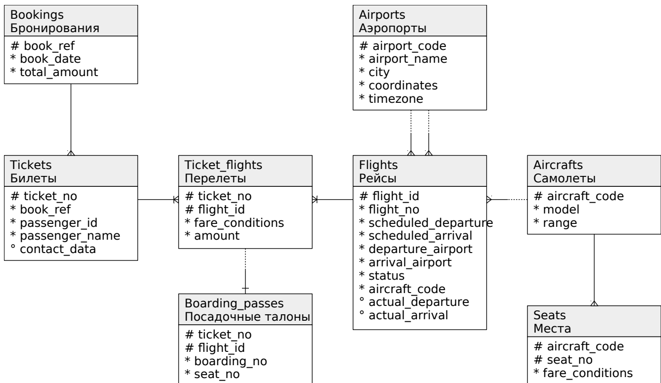
Рисунок 17.2. Исходная схема базы данных
