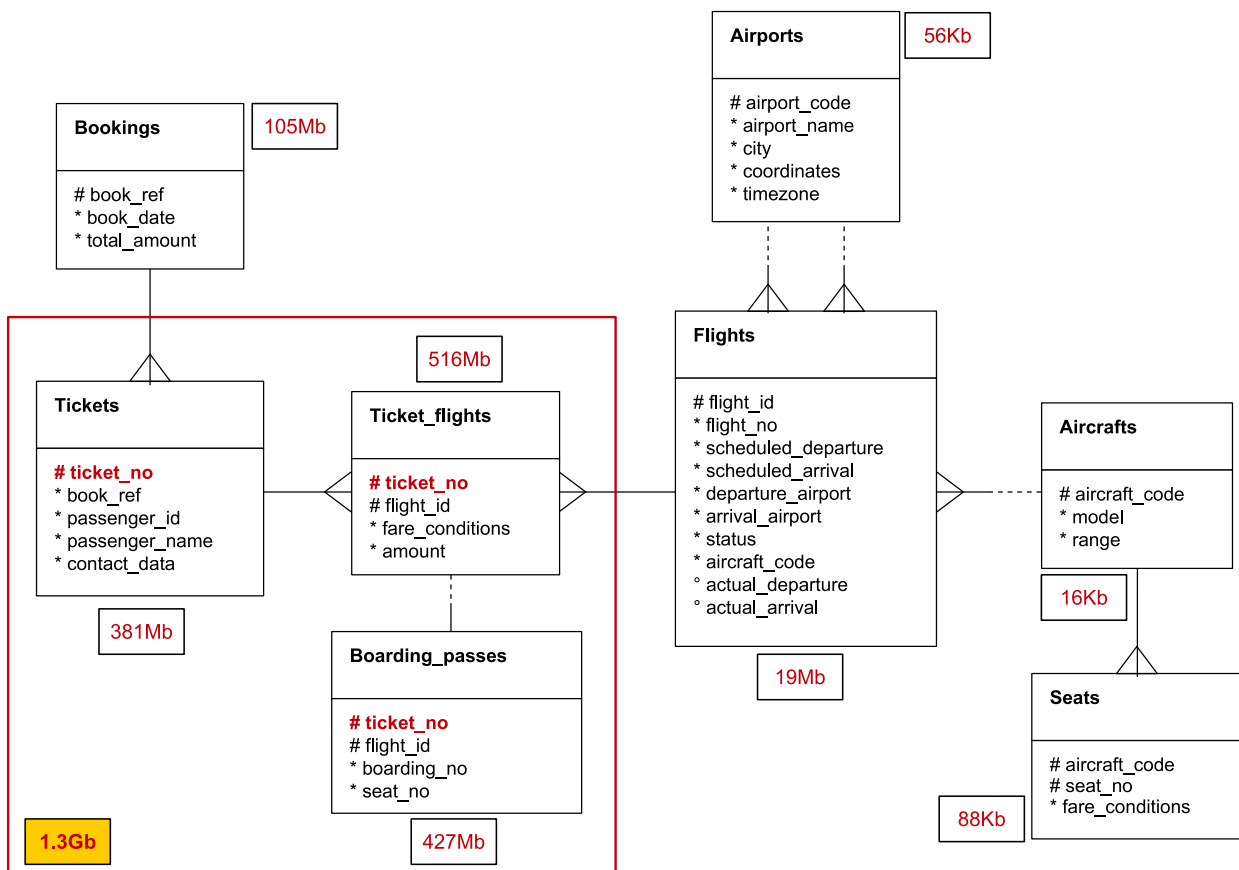
Рисунок 17.3. Схема наивного подхода
