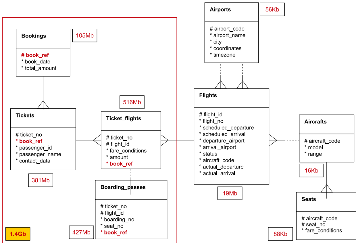
Рисунок 17.4. Изменение исходной схемы
