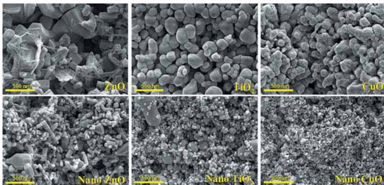
Joonis 5. Skaneeriva elektronmikroskoobi fotod ZnO, TiO 2 ja CuO nano- ja tava suuruses osakestest [8]
