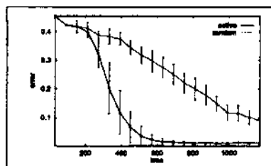
Fig. 12. Estimation error
