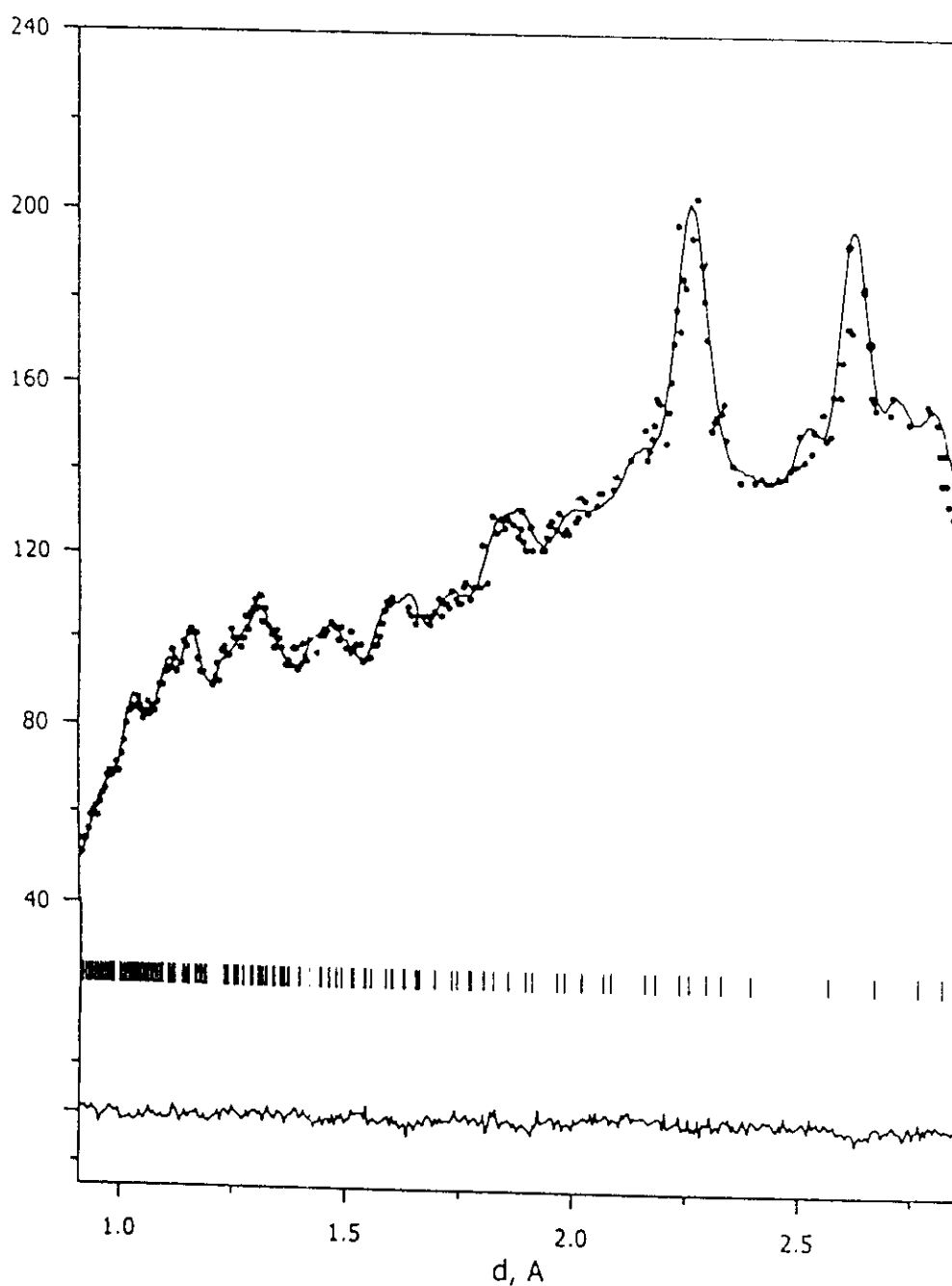
Рис.1. Дифракционный спектр позвоночной кости крупного рогатого скота . (Фаза: \text{Ca}_5[\text{PO}_4]_3(\text{OH}, \text{F}, \text{Cl}) ). Точки — исходный спектр, линия — расчет, внизу - их разность и расчетные положения пиков
