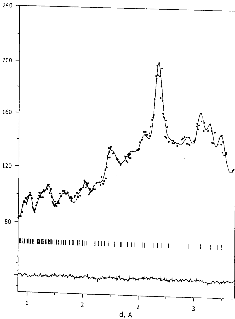
Рис.2. Дифракционный спектр плечевой кости овцы . (Фаза: \text{Ca}_5[\text{PO}_4]_3(\text{OH}, \text{F}, \text{Cl}) ). Точки — исходный спектр, линия — расчет, внизу - их разность и расчетные положения пиков
