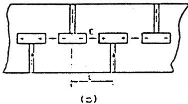
Fig. 46. Interdigital line.
