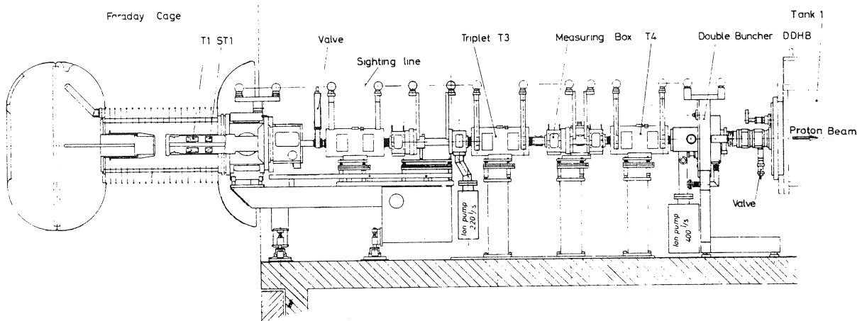
Fig. 2 Preinjector and LEBT
