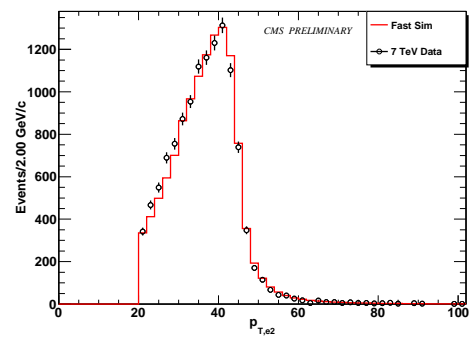
(d) Sub-leading Electron p_T
