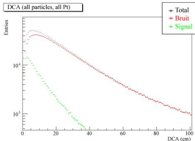
FIG. 9.1 – Distribution en DCA du signal, du bruit, et totale pour toutes les traces reconstruites dans le spectromètre à muons sans le système de déclenchement.
