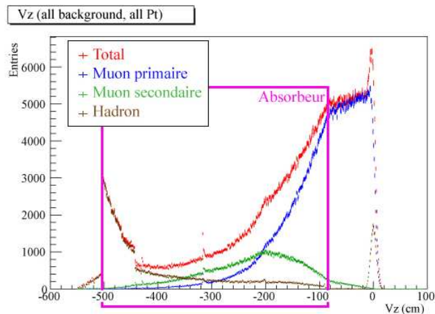
FIG. 9.8 – Distribution de la position V_z (en cm) suivant l'axe Oz des vertex de formation des particules de bruit.
