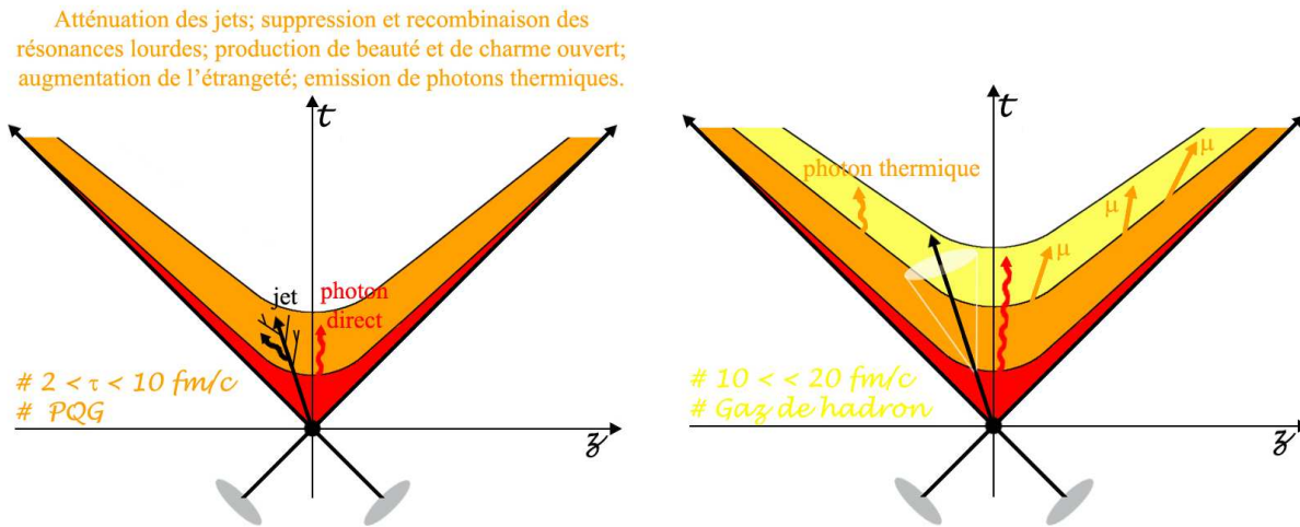
FIG. 2.12 – Deuxième étape de la collision dans le cas d’une collision d’ions lourds. De la même manière les chiffres ne sont que des ordres de grandeurs, reflets des différentes échelles de temps.
