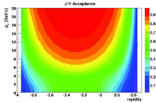
(a) Acceptance fonction de l'impulsion transverse p_t [GeV/c] et de la rapidité y .
