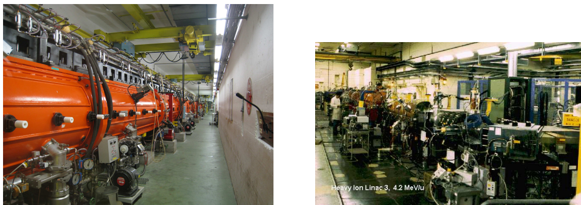
FIG. 2.5 – Photo de LINAC 2 à gauche et LINAC 3 à droite.
