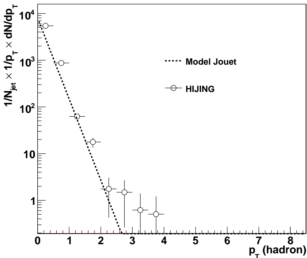
FIG. 1.15 – Spectre en impulsion transverse des particules du bruit de fond pour notre modèle simple (trait pointillé) et pour des simulations effectuées avec HIJING (symboles ronds ouverts).
