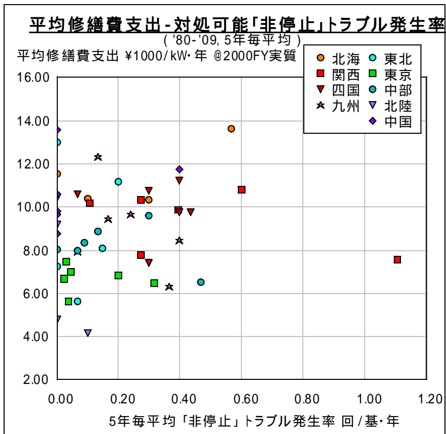
[図4-2-2-4. 平均修繕費支出と対処可能「非停止」トラブル発生率(5年毎平均,一般電気事業者別)]
