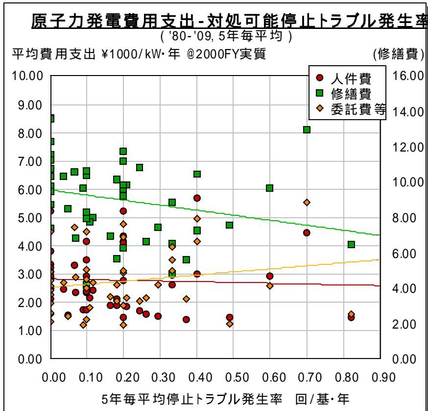
[図4-2-1-2. 原子力発電費用支出と対処可能停止トラブル発生率の相関 (5年毎平均)]
