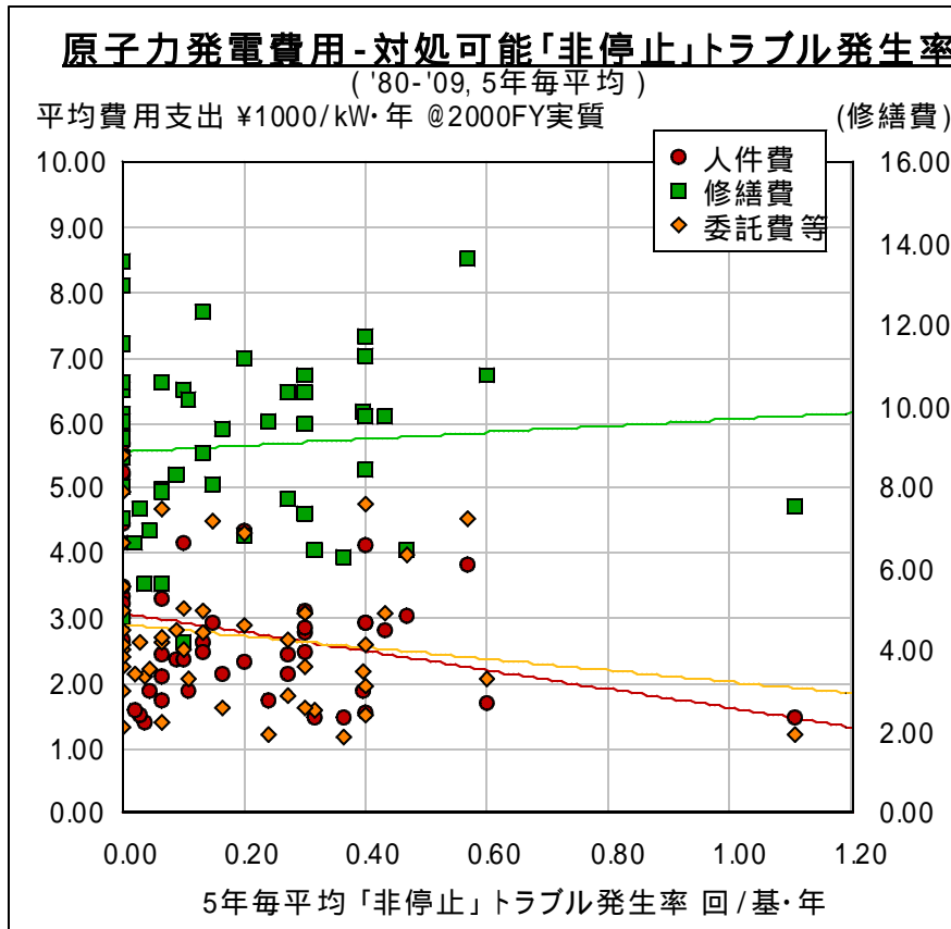
[図4-2-2-2. 原子力発電費用支出と対処可能「非停止」トラブル発生率相関 (5年毎平均)]
