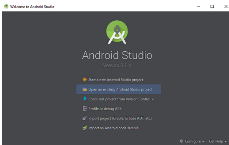
図 2.5.7 Open project
