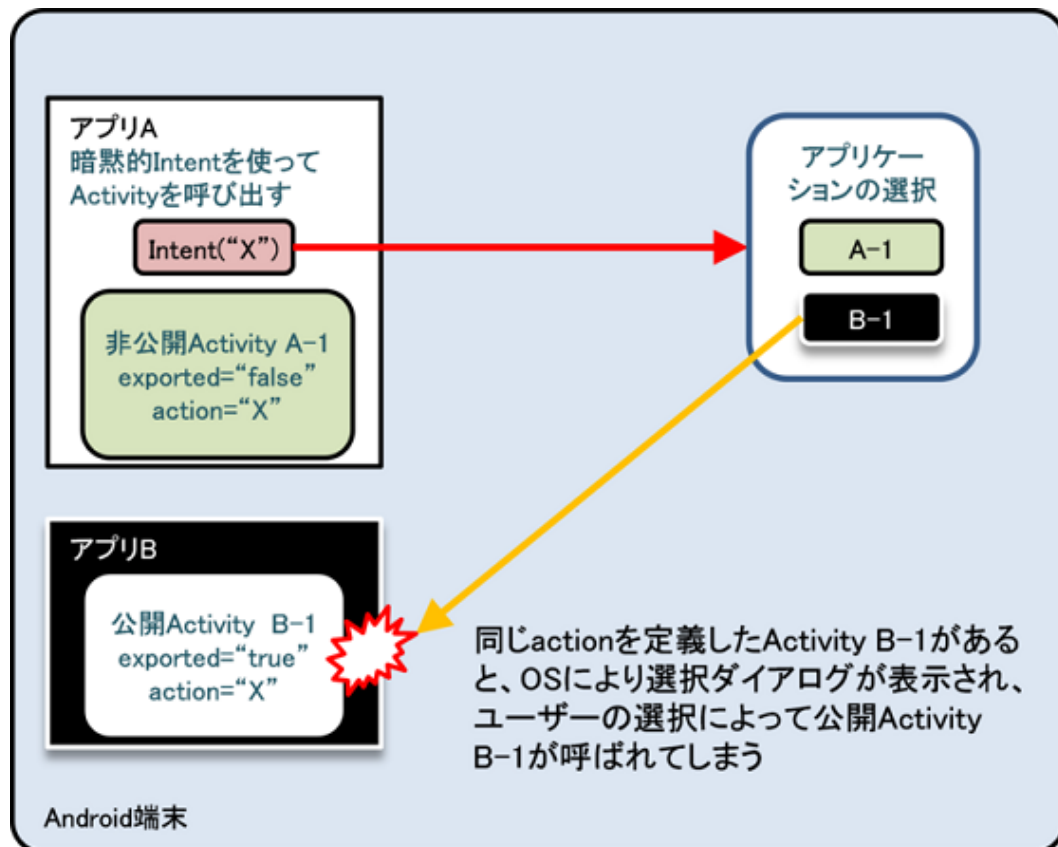
図 4.1.5 意図しない動作の例
