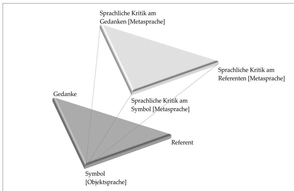
Abb. 1: Modifikation des semiotischen Dreiecks nach Ogden/Richards (1974: 18)
