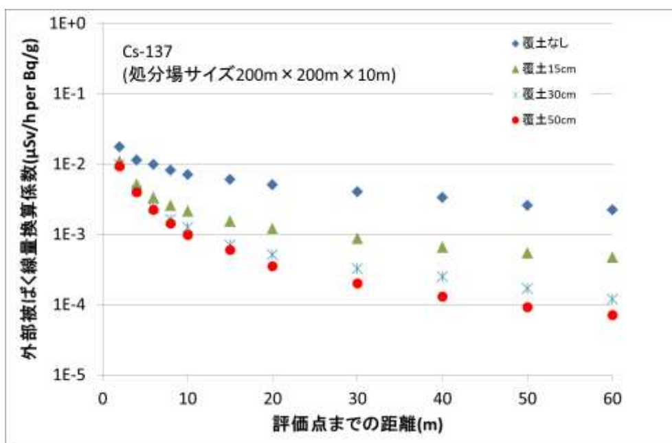
図4 Cs-137 線量換算係数の即日覆土厚と評価点までの距離との関係（災害廃棄物直接埋設処分場 200m×200m×10m，敷均し面積 15m×15m）
