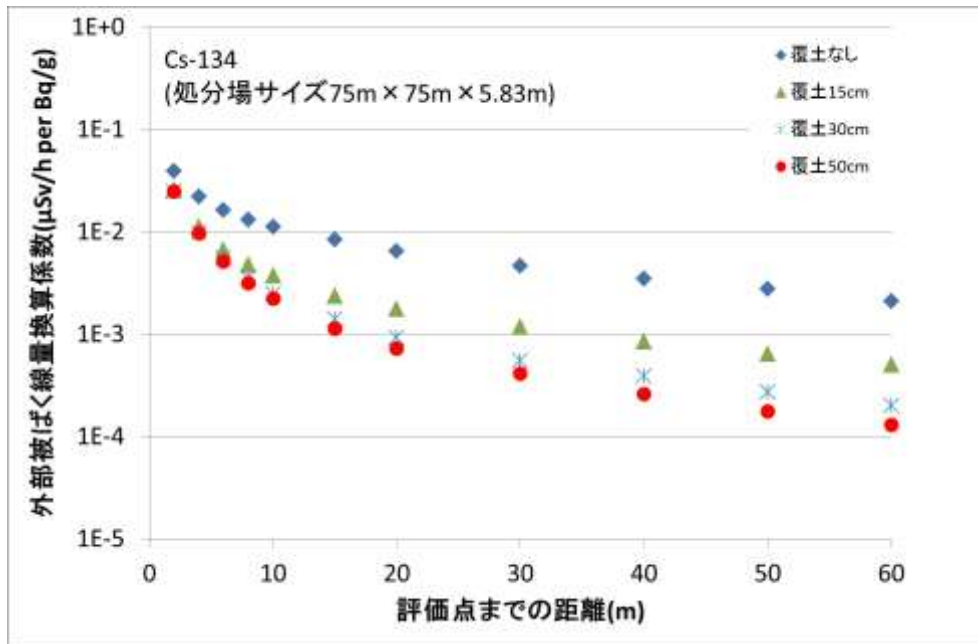
図1 Cs-134 線量換算係数の即日覆土厚と評価点までの距離との関係 (焼却灰埋設処分場 75m×75m×5.83m, 敷均し面積 12m×12m)
