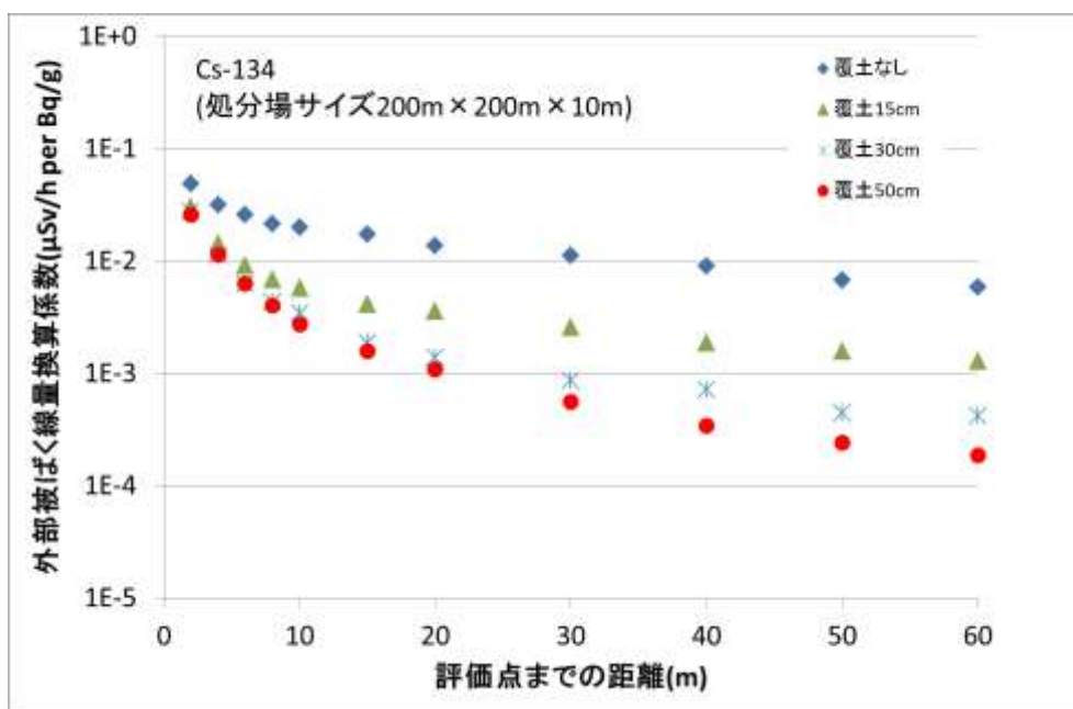
図3 Cs-134 線量換算係数の即日覆土厚と評価点までの距離との関係（災害廃棄物直接埋設処分場 200m×200m×10m，敷均し面積 15m×15m）
