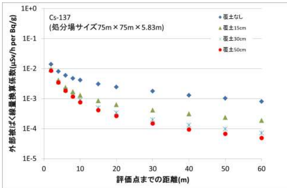
図2 Cs-137 線量換算係数の即日覆土厚と評価点までの距離との関係 (焼却灰埋設処分場 75m×75m×5.83m, 敷均し面積 12m×12m)
