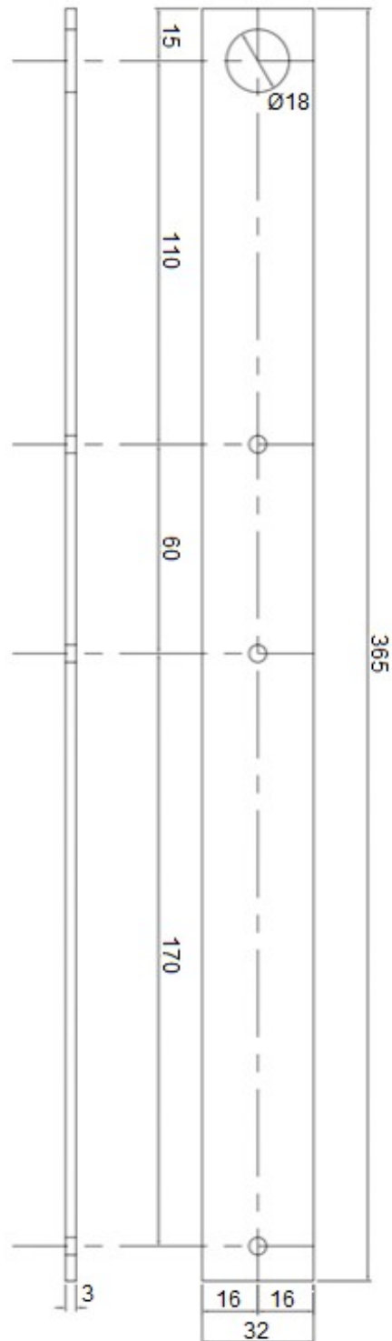
Figura 1 - Suporte de identificação tipo 1
