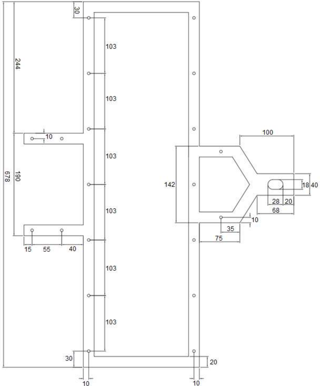
Figura 3 - Suporte de identificação tipo 3
