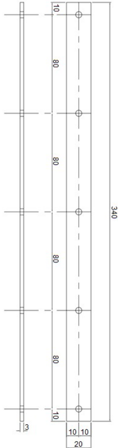
Figura 2 - Suporte de identificação tipo 2
