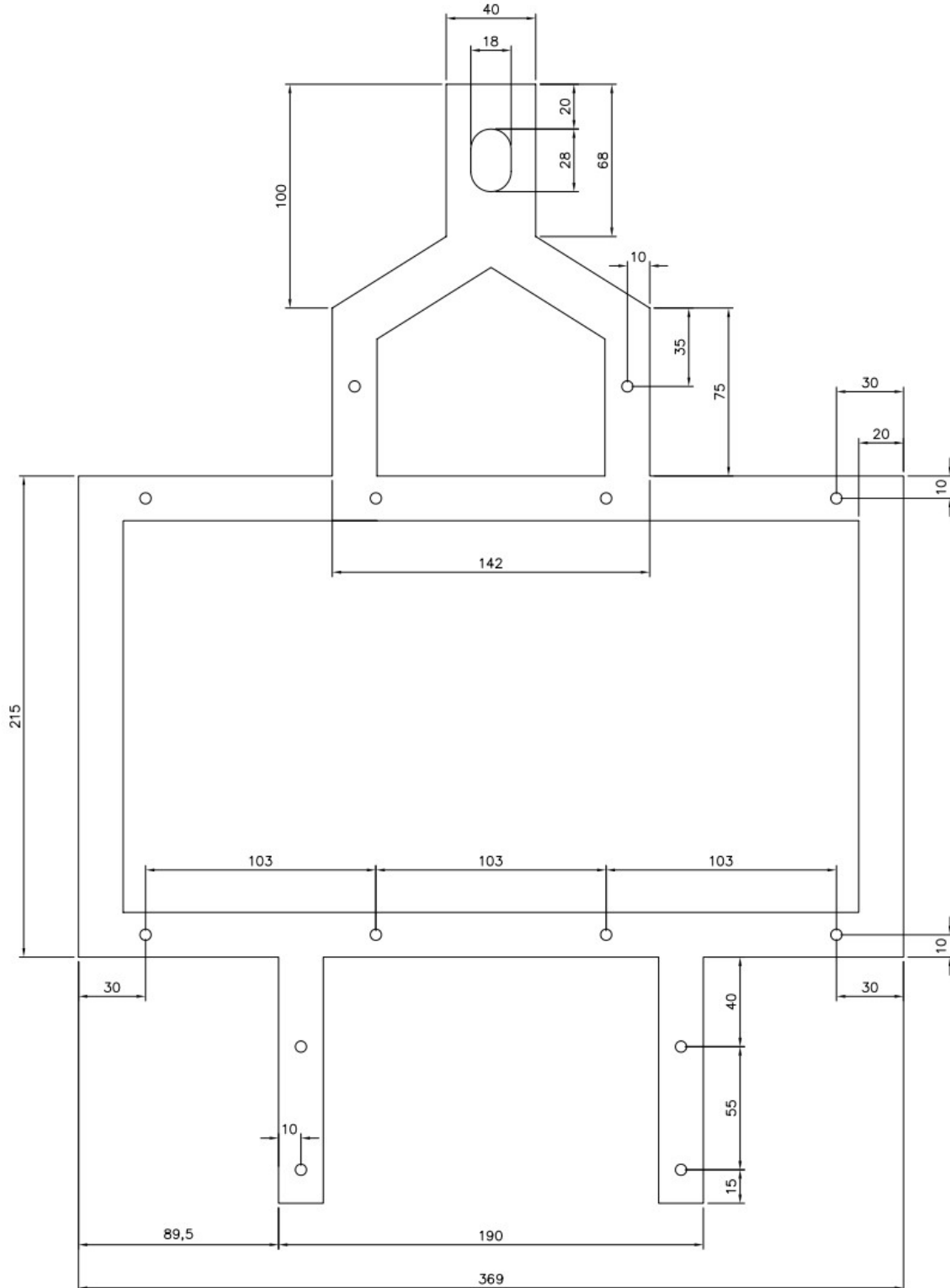
Figura 4 - Suporte de identificação tipo 4
