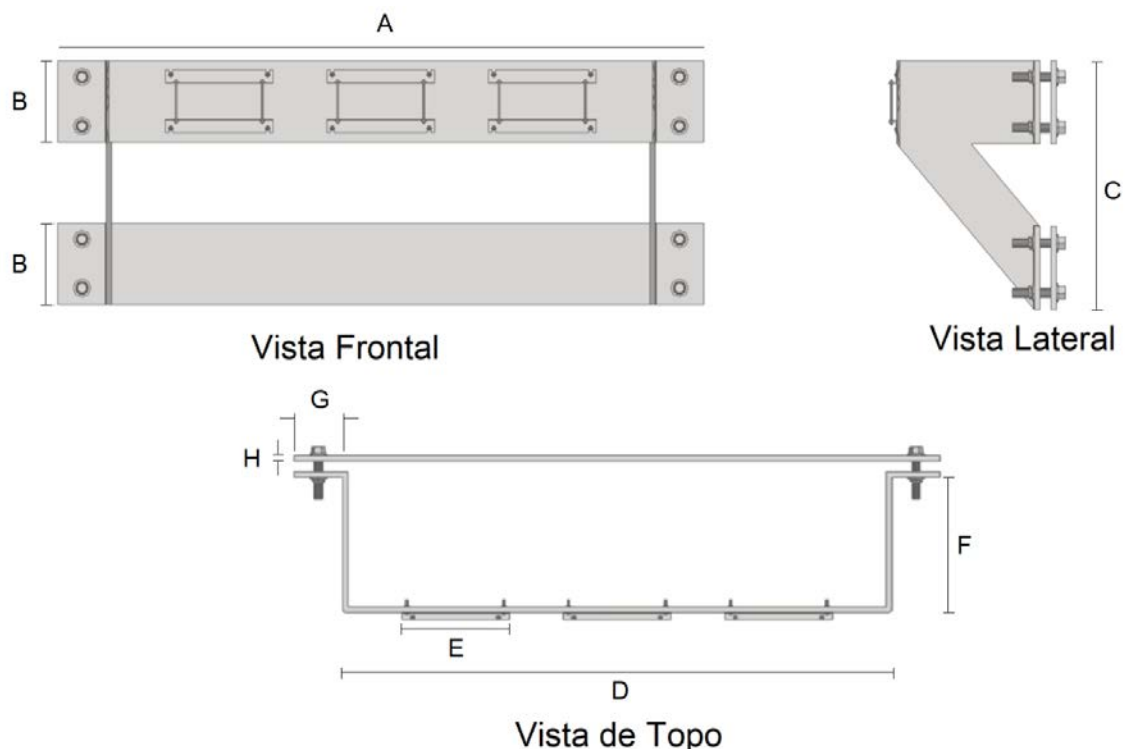
Figura 2 - Vistas do Suporte Horizontal
