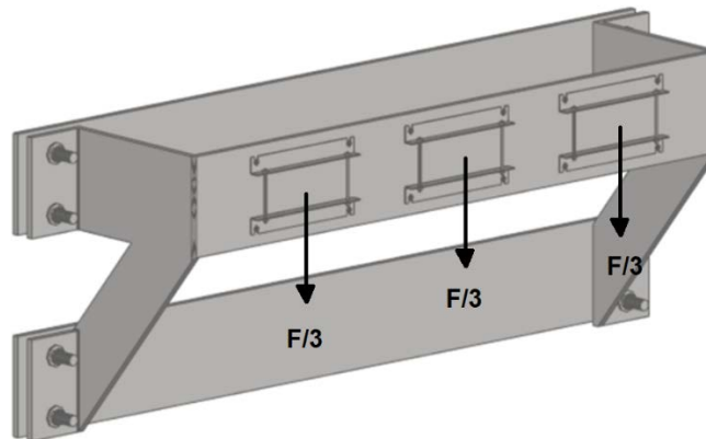
Figura 3 – Detalhe para execução do ensaio
