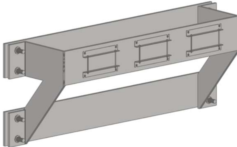
Figura 1 - Suporte Horizontal para Transformador de Corrente
