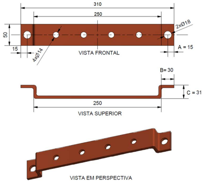
Figura 1 - Barra de cobre para aterramento
