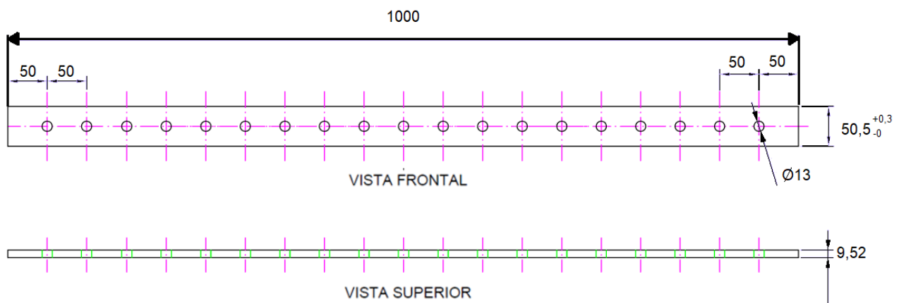
Figura 2 - Barra para interligação de cabos terra em câmaras transformadoras
