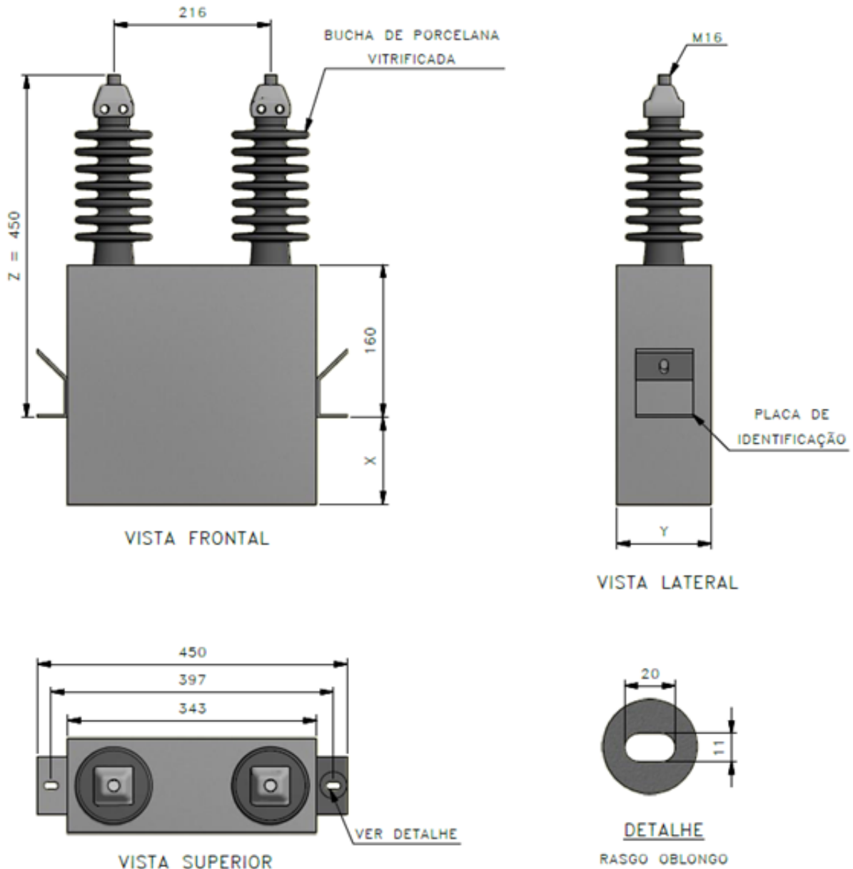
Figura 1 - Capacitor de Potência em Derivação
