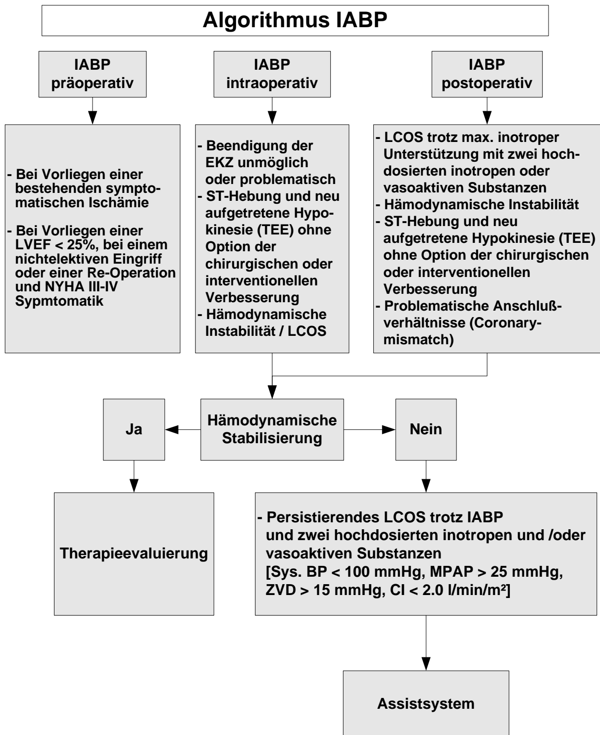
Abbildung 7: Algorithmus IABP
