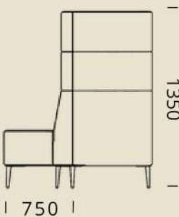
OAS-TB-45CAV
