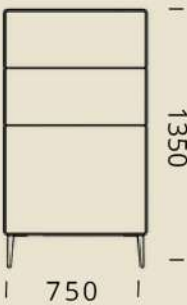
OAS-TB-3SLR
