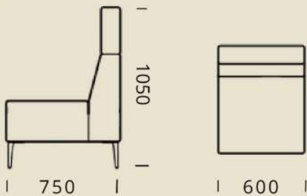
OAS-MB-1SST
