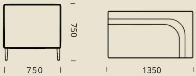
OAS-SB-2SR
