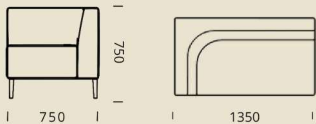
OAS-SB-2SL
