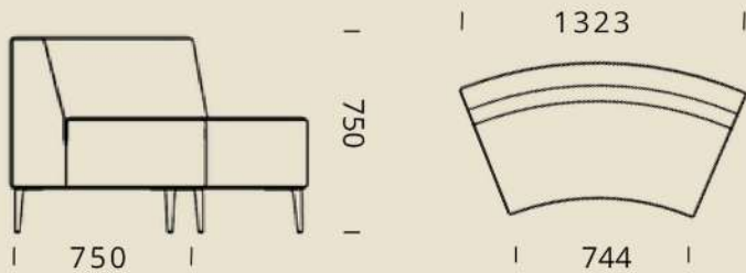
OAS-SB-45CAV
