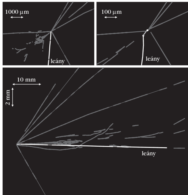
6. ábra. Az OPERA-kísérlet által azonosított esemény tau-neutrínó keletkezésével. Ez annak bizonyítéka, hogy a müon-neutrínó valóban át tud alakulni tau-neutrínóvá [5].
