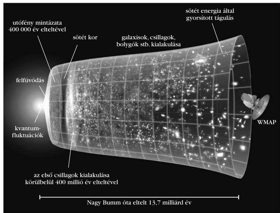
3. ábra. A Világegyetem története a kozmológia jelenlegi állása szerint. Időrendben: Ősrobbanás, felfúvódás, sugárzás, átlátszóság, galaxisok kialakulása, napjaink gyorsuló tágulása.
