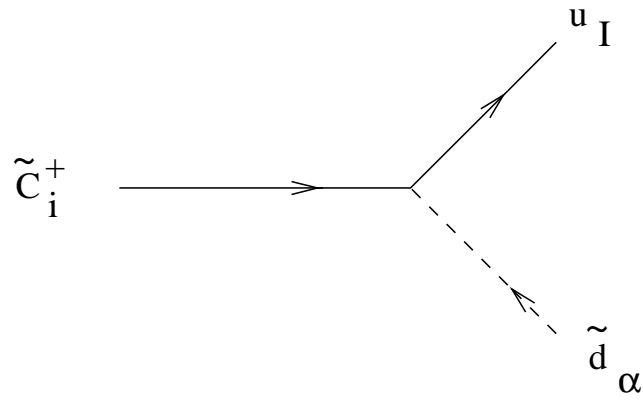
Figure 10: \frac{g}{2m_W \cos} (V^{CKM})_{IJ} (S^{CKM})_{DL}^J U_{i1} \not{P} + \frac{g_2}{2m_W \cos} (V^{CKM})_{IJ} (S^{CKM})_{DR}^J m_J^d U_{i2} \not{P} + \frac{g_2}{2m_W \sin} (V^{CKM})_{IJ} (S^{CKM})_{DL}^J m_I^u V_{i2} \not{P}
