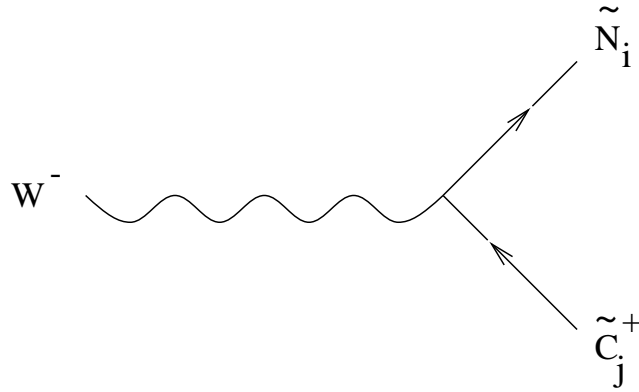
Figure 18: g_2 (O_{ij}^L P_L + O_{ij}^R P_R)
