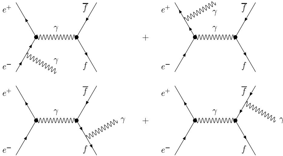
Fig. 12: Bremsstrahlung process e^+e^- \rightarrow f\bar{f}\gamma .
