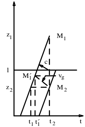
Fig. 2. Backward wake
