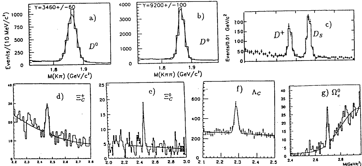
Fig. 4. Charmed hadron invariant mass plots from E-687. a) D^0 , b) D^+ , c) D_S , d) \Xi_C^+ , e) \Xi_C^0 , f) \Lambda_C , g) \Omega_C^0
