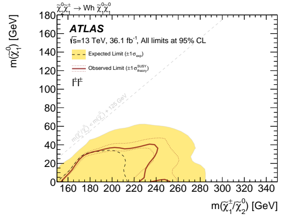
(d) \ell^+\ell^-
