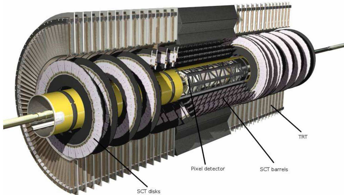
Abbildung 3.3: Schematische Darstellung des Inneren Detektors.
