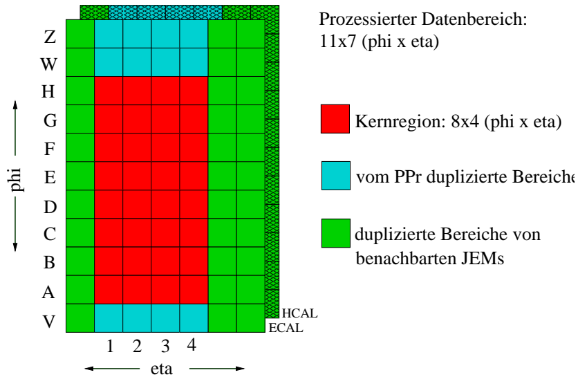
Abbildung 5.1: Prozessierter Datenbereich in \phi und \eta eines JEM.
