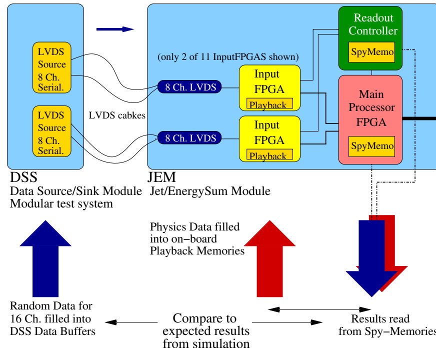
Abbildung 5.12: Standalone Tests des JEM im DSS/Spy-Modus.
