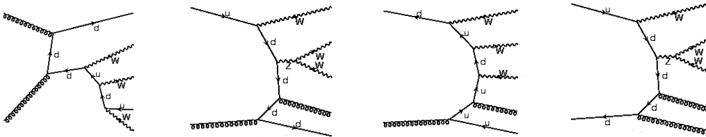
Abbildung 7.3: Beispiele von Feynmangraphen für pp \rightarrow W^+W^+W^-jj ( gg \rightarrow W^+W^+W^-ud , ug \rightarrow W^+W^+W^-dg , \bar{d}g \rightarrow W^+W^+W^-ug und u\bar{d} \rightarrow W^+W^+W^-gg ).
