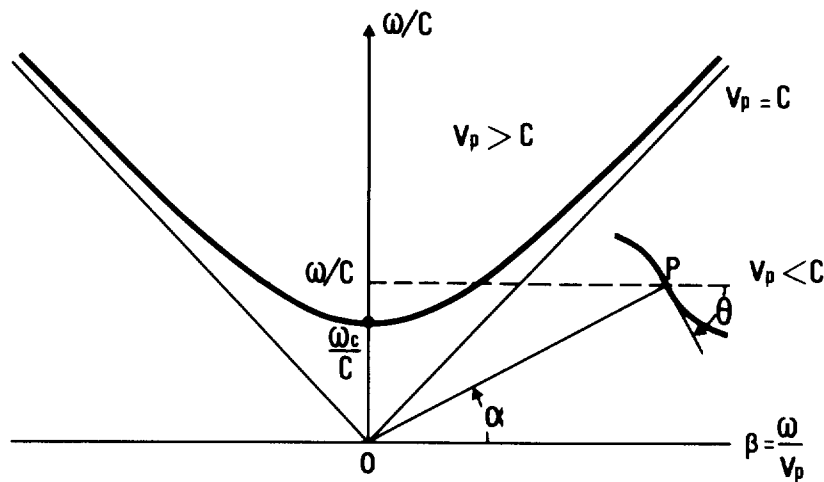
Fig. 16 - Brillouin diagram
