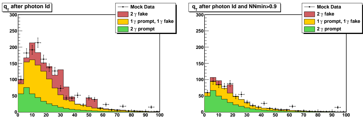
FIG. 8.8 – Distribution de l'impulsion transverse q_T du système diphoton dans les données artificielles et la simulation après identification des photons (à gauche) par isolation puis coupure sur le réseau de neurone (à droite).
