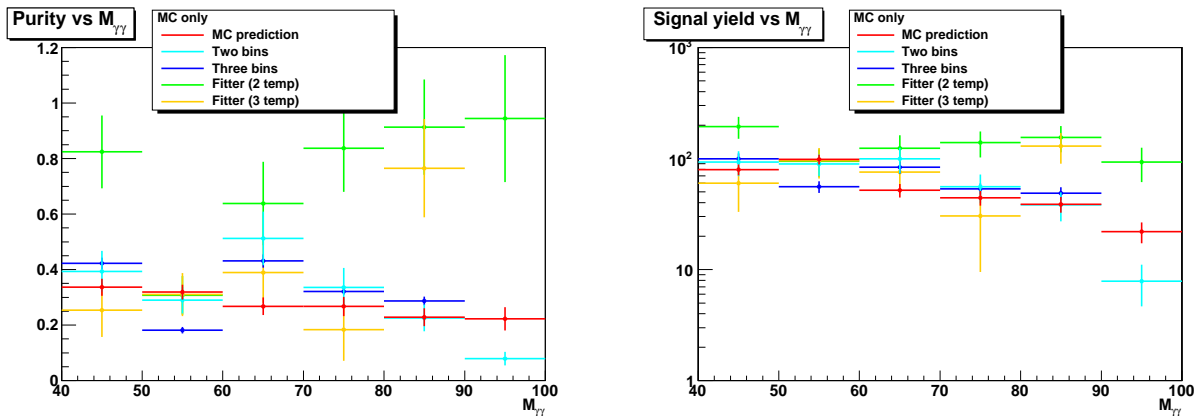
FIG. 8.7 – Pureté et nombre d'évènements de signal en fonction de la masse invariante \gamma\gamma dans les données artificielles, estimées par quatre méthodes templates et dans la simulation.
