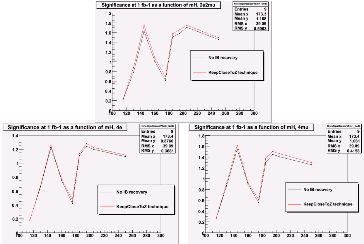
FIG. 4.22 – Significance obtenue avec 1 fb^{-1} de luminosité intégrée et une énergie de 10 TeV dans le centre de masse, dans le canal 2e2\mu (en haut), 4e (à gauche) et 4\mu (à droite) sans récupération de photons FSR (en noir) et avec récupération par la méthode “KeepCloseToZ” (en rouge), en fonction de la masse du boson de Higgs.
