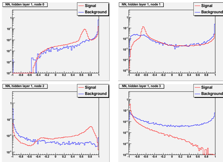
FIG. 5.18 – Distributions de sorties de chacune des quatre neurones de la première couche cachée, pour le réseau de neurone entraîné avec les variables de forme du cluster.
