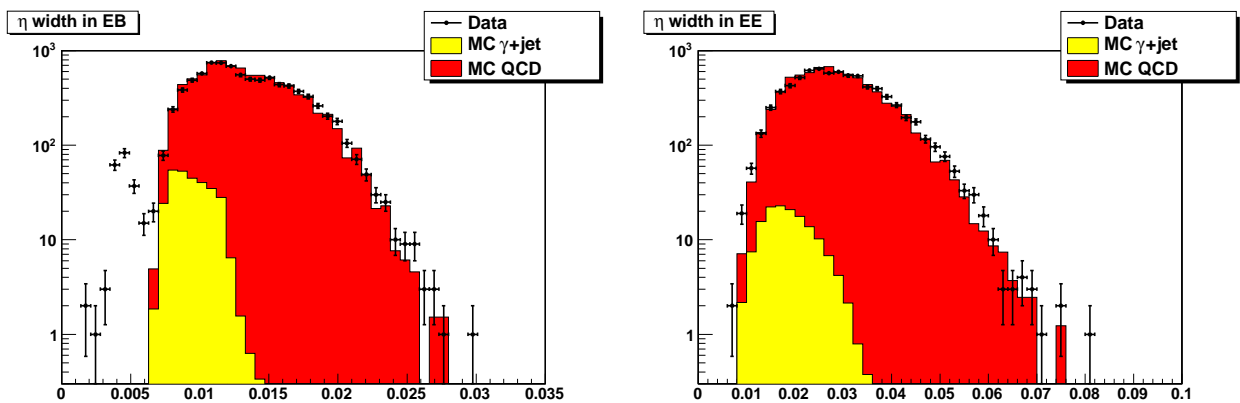
FIG. 5.39 – Distribution de la variable d'entrée \sigma_\eta dans les données et la simulation, dans le tonneau (à gauche) et les bouchons (à droite).
