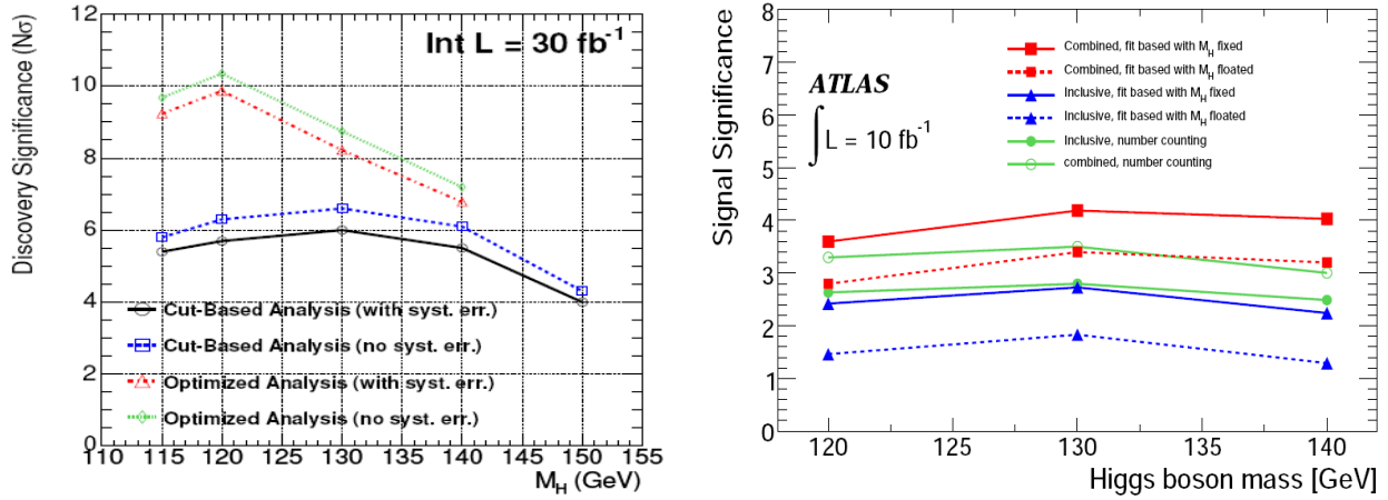
FIG. 2.16 – Significane pour l’observation du boson de Higgs avec une énergie dans le centre de masse de 14 TeV pour une luminosité intégrée de 10 fb^{-1} pour ATLAS (à droite), et 30 fb^{-1} pour CMS (à gauche), dans le canal H \rightarrow \gamma\gamma .
