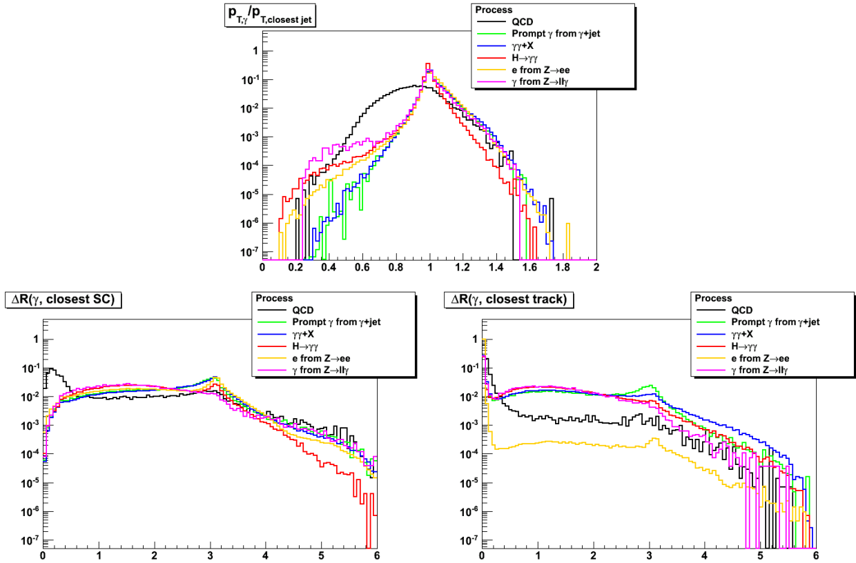
FIG. 5.31 – Distribution des variable d’environnement \frac{p_{T,\gamma}}{p_{T,closestjet}} , \Delta R(\gamma,closestSC) et \Delta R(\gamma,closesttrack) pour les électrons de Z \rightarrow ee et les photons prompts de Z \rightarrow ll\gamma comparées au bruit de fond et aux autres processus de signal.
