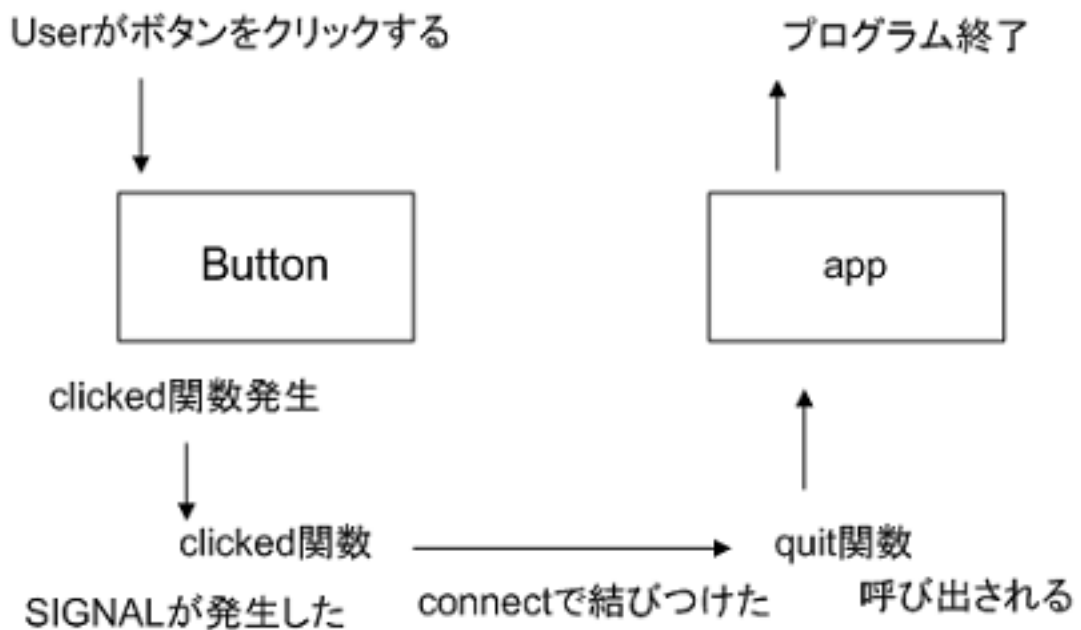
図 3.2: Signal/Slot のイメージ図
