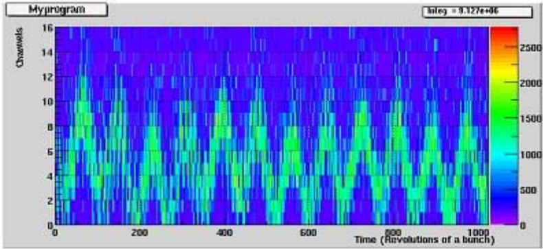
Рис. 7. Эволюция пучка во времени в присутствии фазовых колебаний. По вертикальной оси – номер канала (анода), по горизонтальной – время, в единицах оборотов пучка. Амплитуда сигнала в цветовой шкале.
