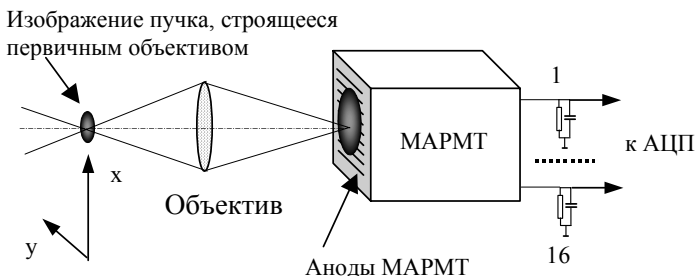
Рис.3. Оптическая схема и расположение анодов ФЭУ относительно пучка.
