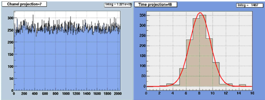
Рис. 8. Проекции распределения. Справа: профиль пучка на 46-м обороте от момента запуска АЦП. Размер одного канала 0.2 мм. Слева: пооборотный сигнал в 7 канале.
