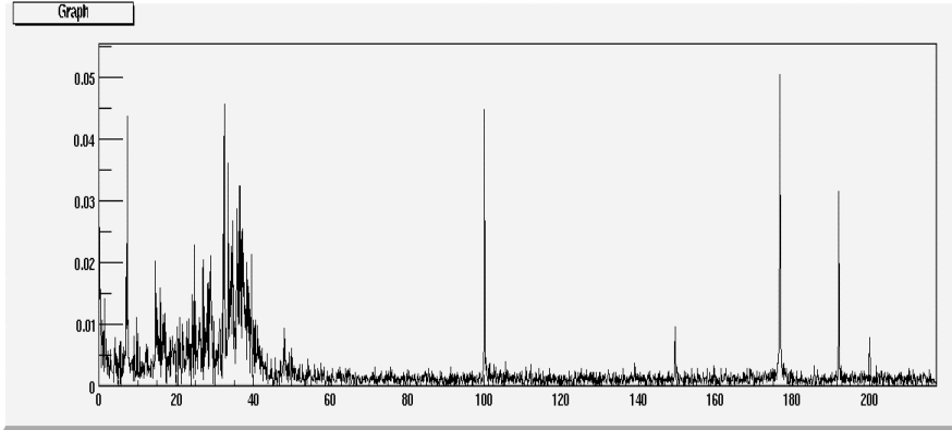
Рис.10. Низкочастотный спектр колебаний пучка.
