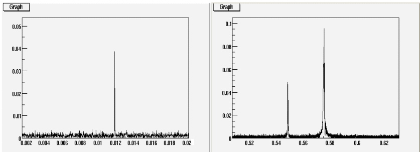
Рис. 9. Частоты колебаний пучка на комплексе ВЭПП-4М.
