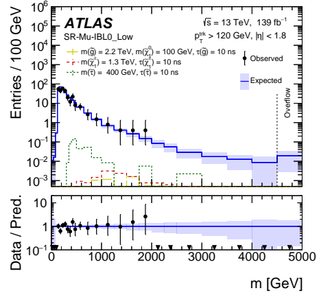
(b) SR-Mu_IBL0_Low
