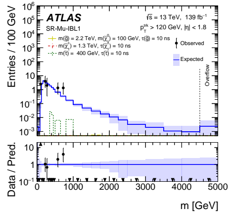
(f) SR-Mu_IBL1
