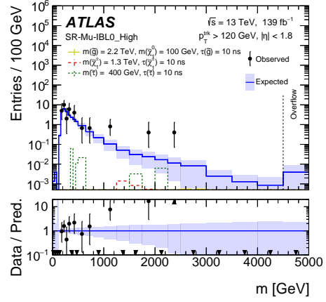
(d) SR-Mu_IBL0_High
