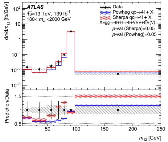
(d) On-shell ZZ region
