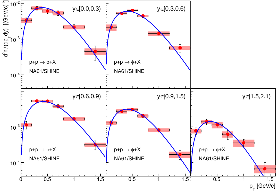
(a) 158 GeV/c
