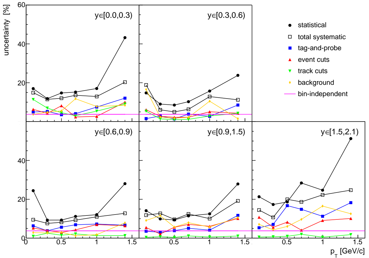
(a) 158 GeV/c
