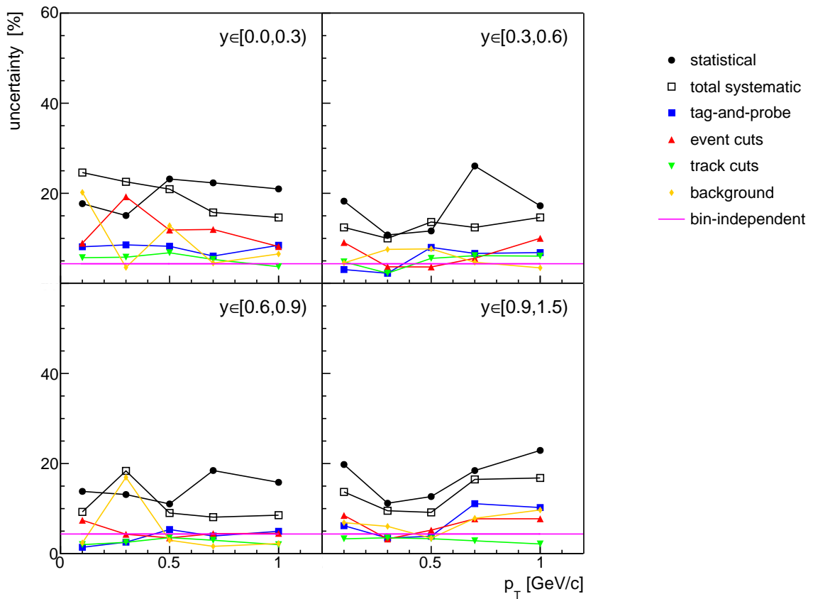
(b) 80 GeV/c
