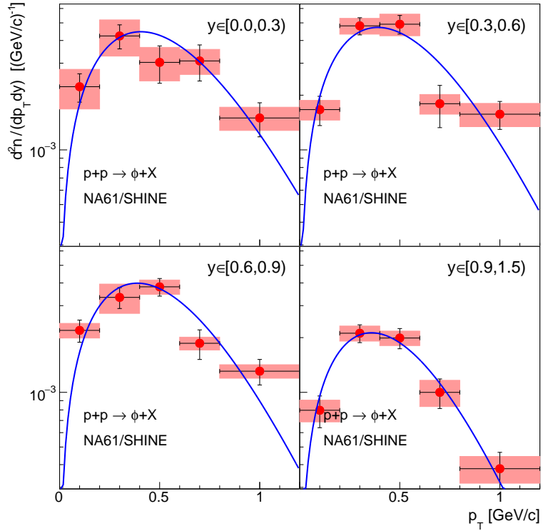
(b) 80 GeV/c
