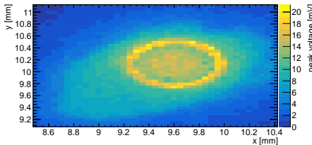
(d) \Phi_{eq} = 3 \cdot 10^{14} \text{ cm}^{-2} , 1677 V
