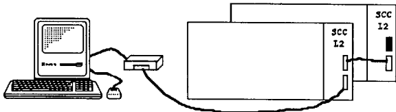
Fig 2 - Macintrotte
